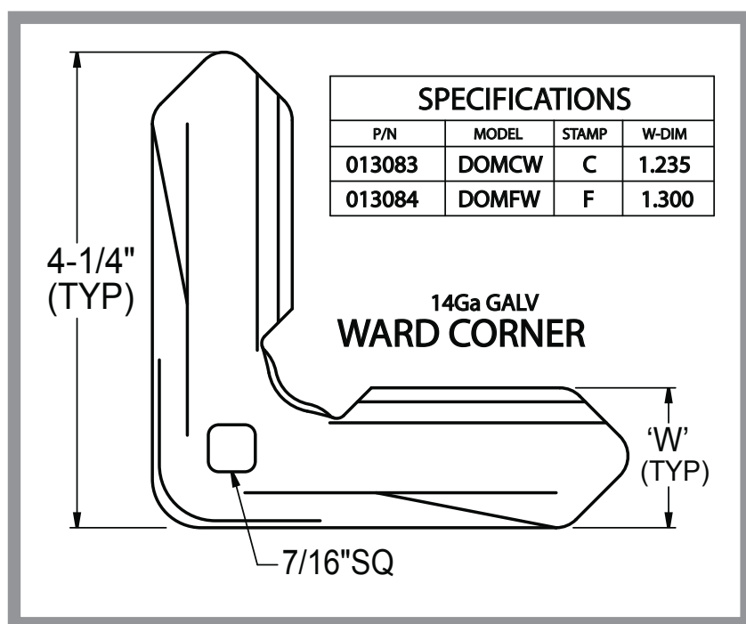
DOMFW Corner
